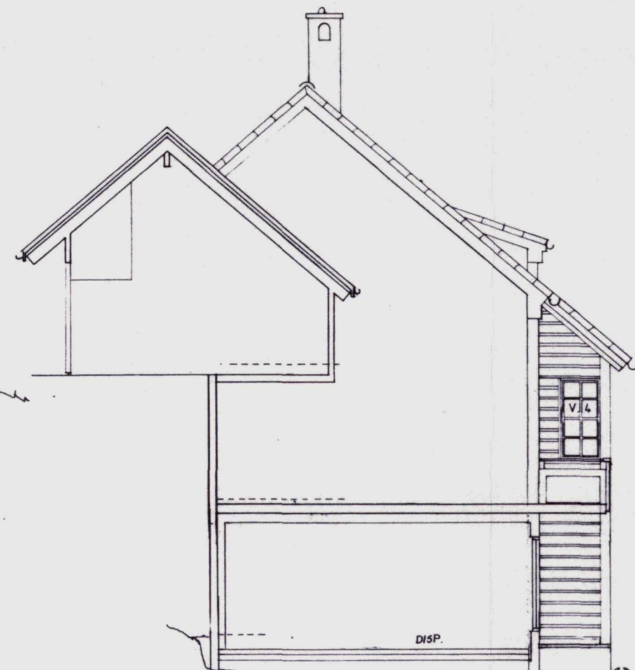
FASADE 2
