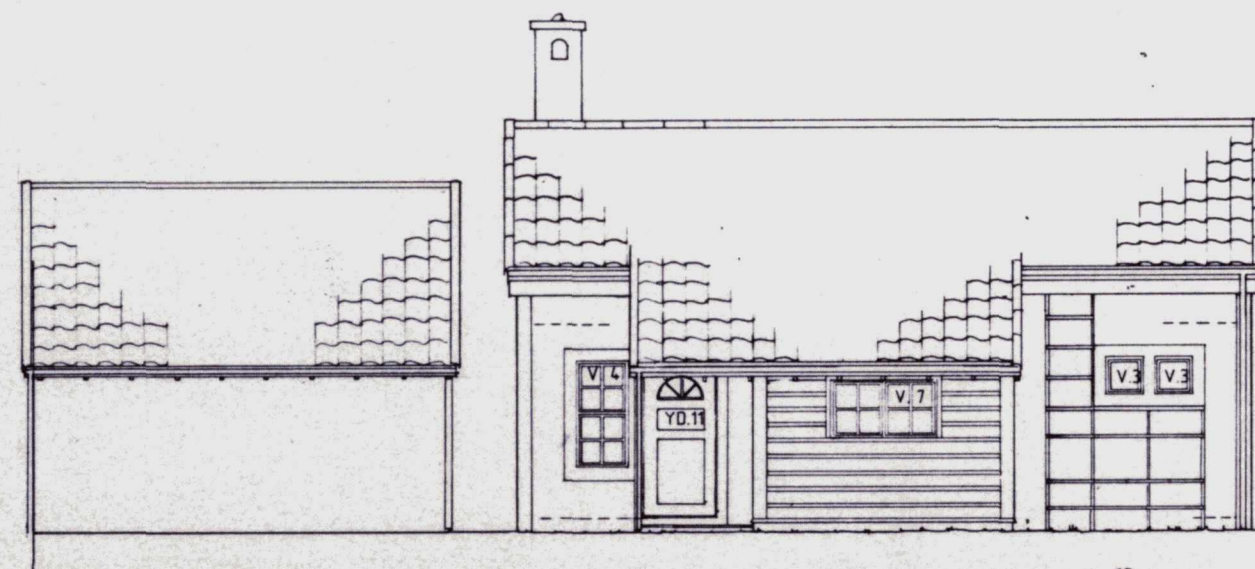
FASADE 3
