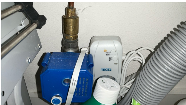
Automatisk lekkasjesikring i kjøkkenskap
