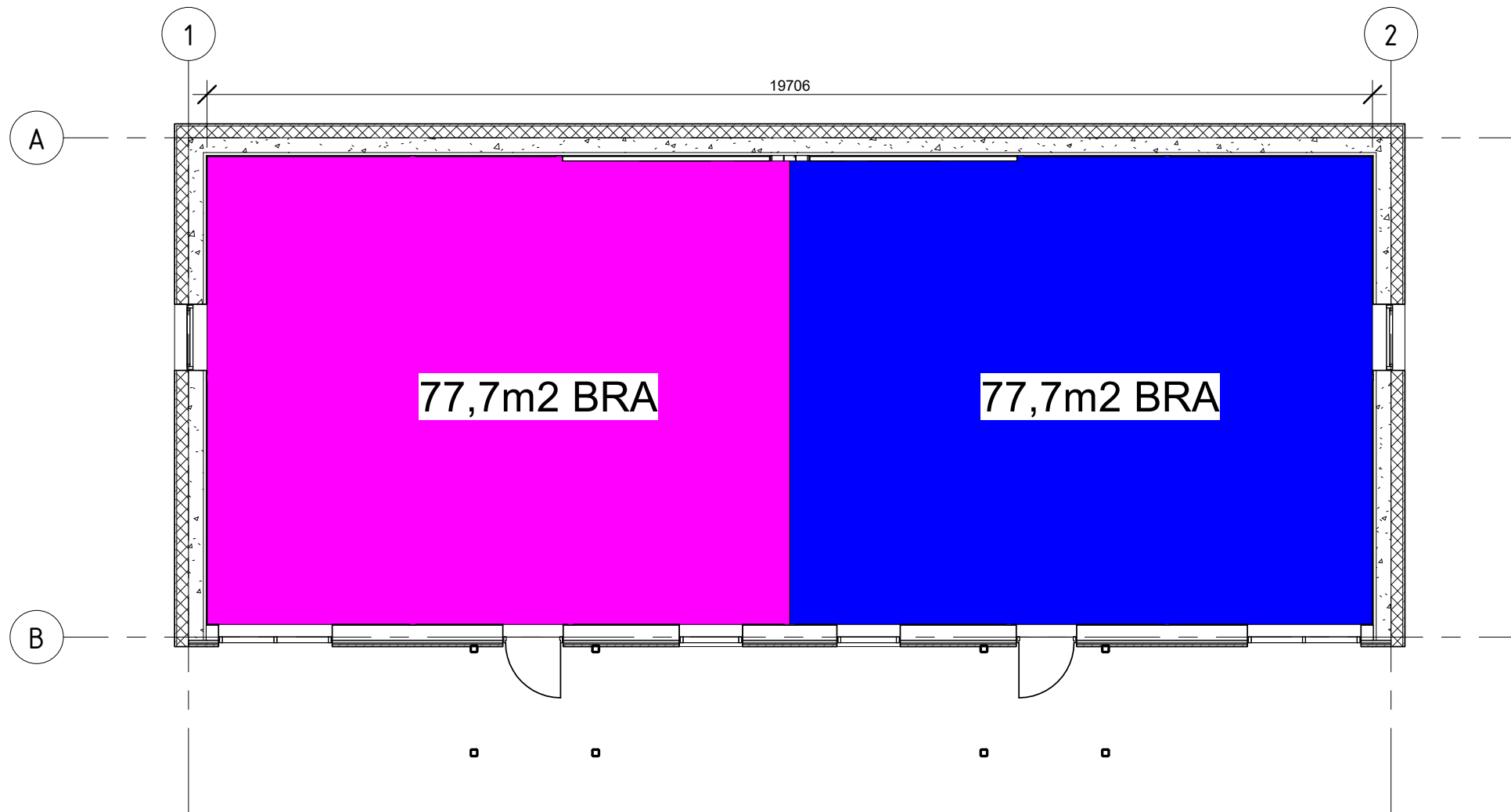
Underetasje BRA 1 : 100
