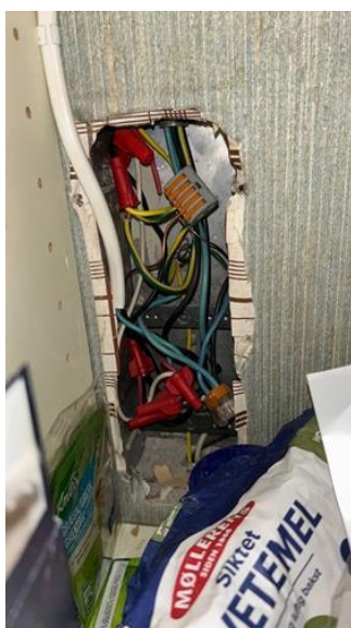
Elektrisk anlegg - [Åpne koblinger i kjøkkenskap]
