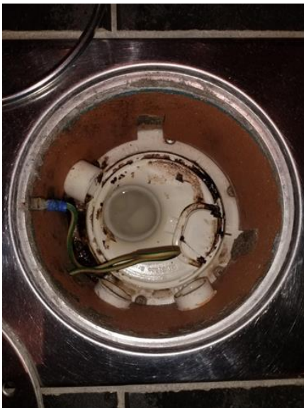
Membran, tettesjikt og overgang til sluk. - [Hovedsluk ]
