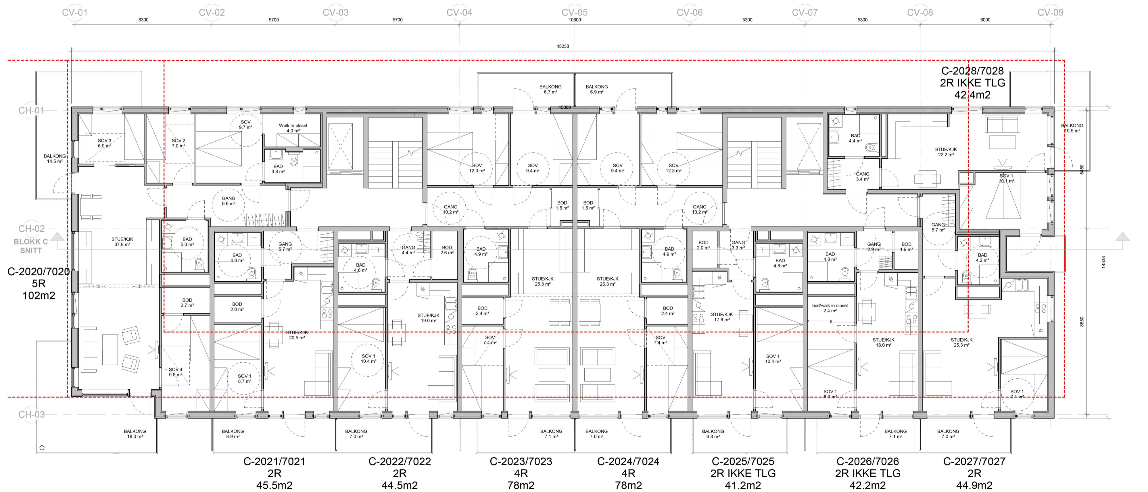
BLOKK C PLAN 02-07 1 : 100
