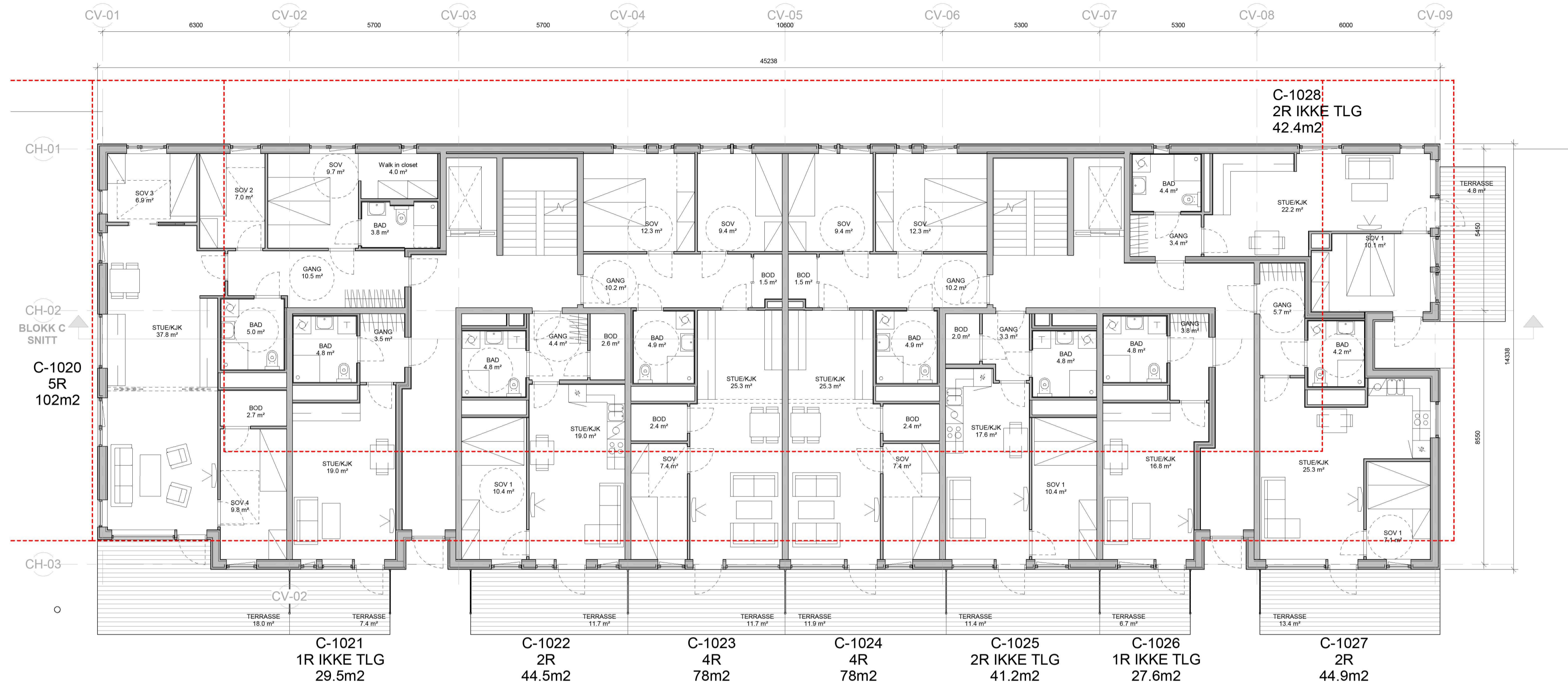
BLOKK C PLAN 01 1 : 100
