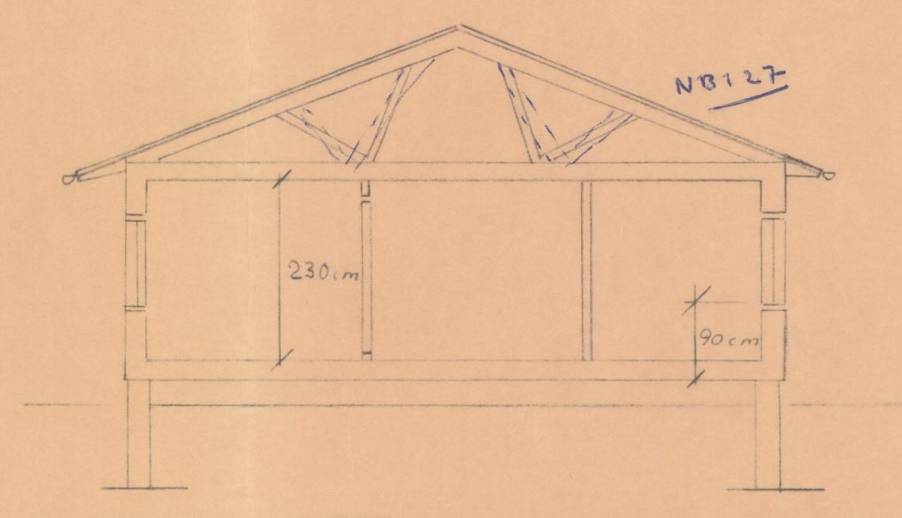
SNITT A-A
