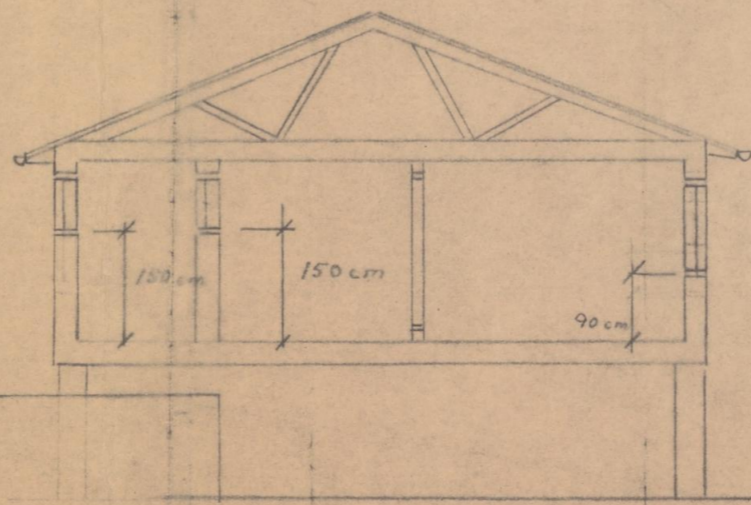
SNITT C-C
