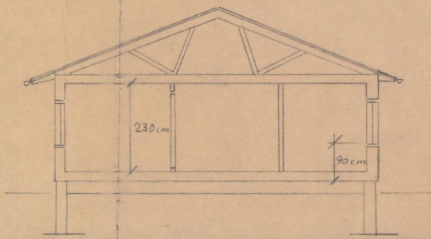
SNITT A-A
