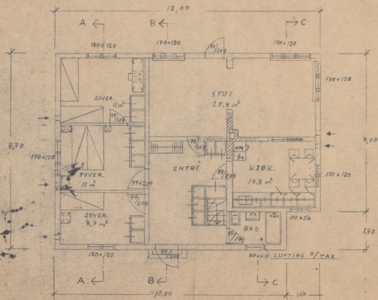
AREAL INNENFOR YTTERVEGGENE 92,5 m 2
