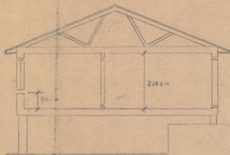
SNITT B-B
