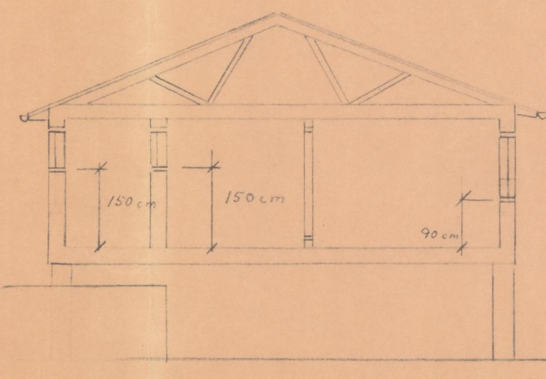
SNITT C-C.
