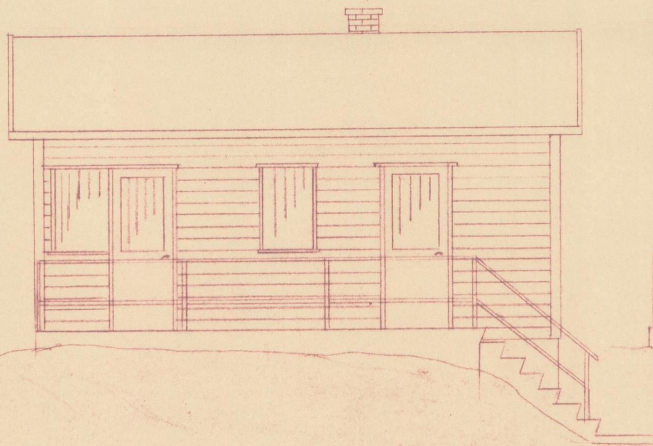
Fasade Øst.
