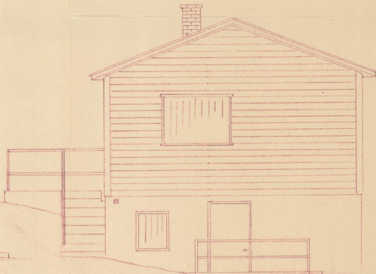
Fasade Nord.
