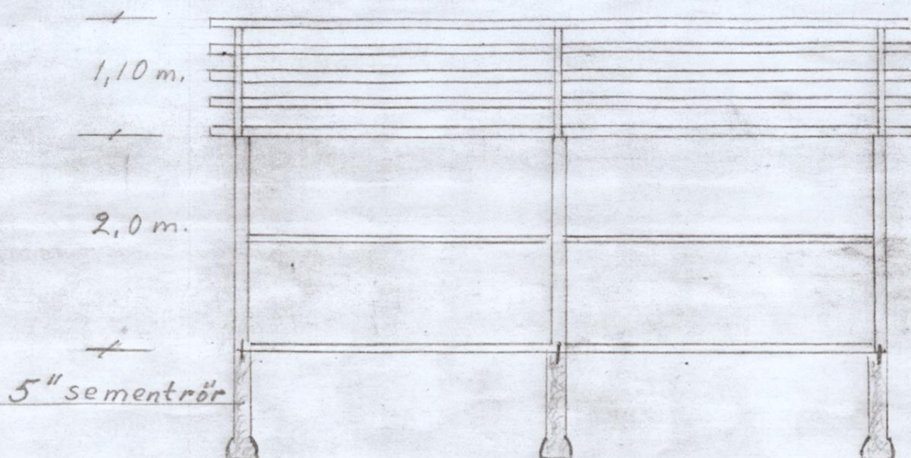
Snitt
