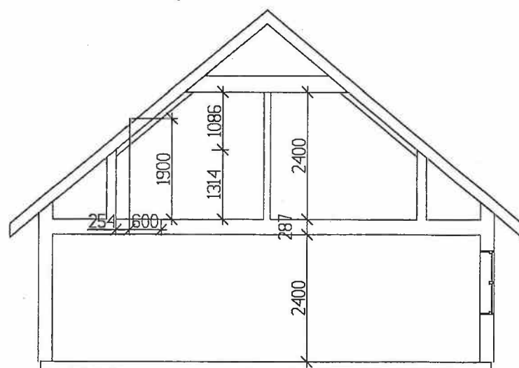
Fasade sydvest
