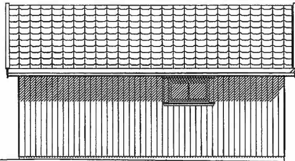
Fasade sydvest
