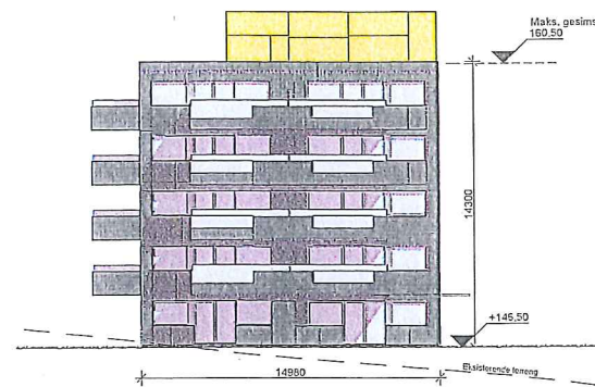
Fasade Sør 1:200
