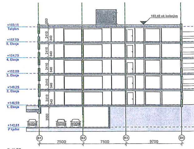
Snitt B2 1:200
