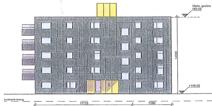
Fasade øst 1:200
