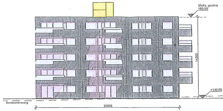
Fasade Vest 1:200
