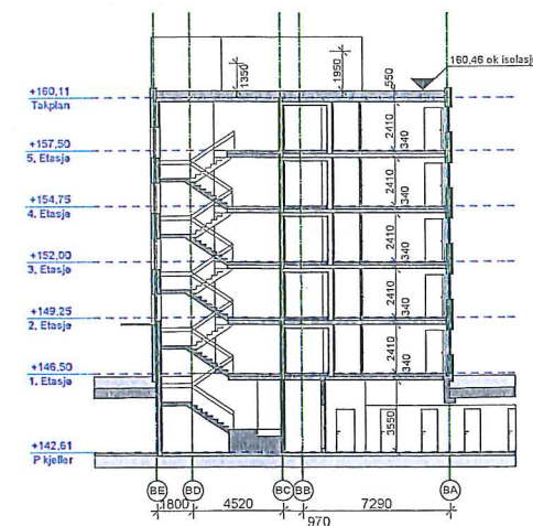
Snitt B1 1:200
