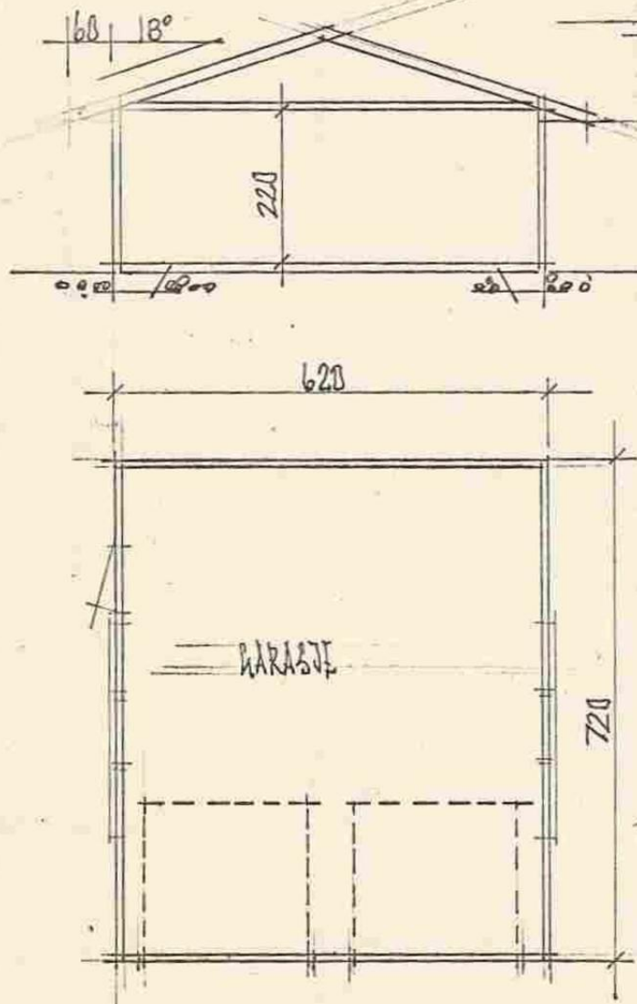
PLAN • SNITT • FASADER AV GARASJE
