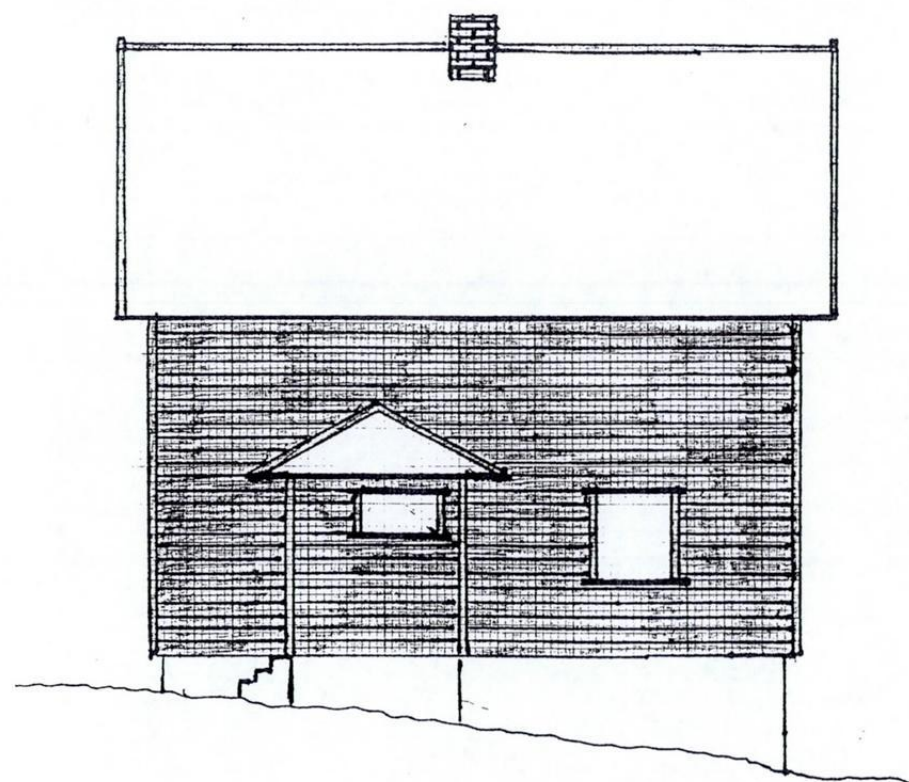
FASADE VEST
