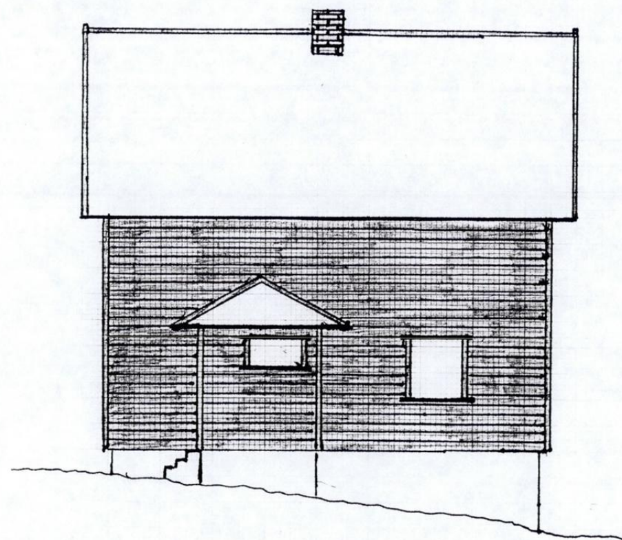
FASADE VEST
