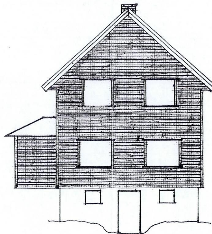
FASADE SYD
