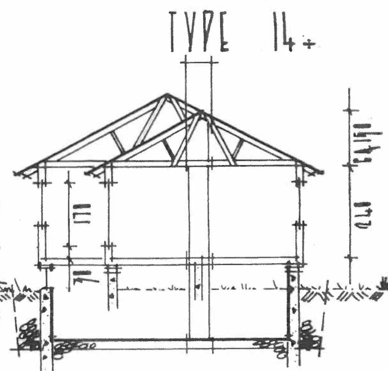
TVÆRSNITT
