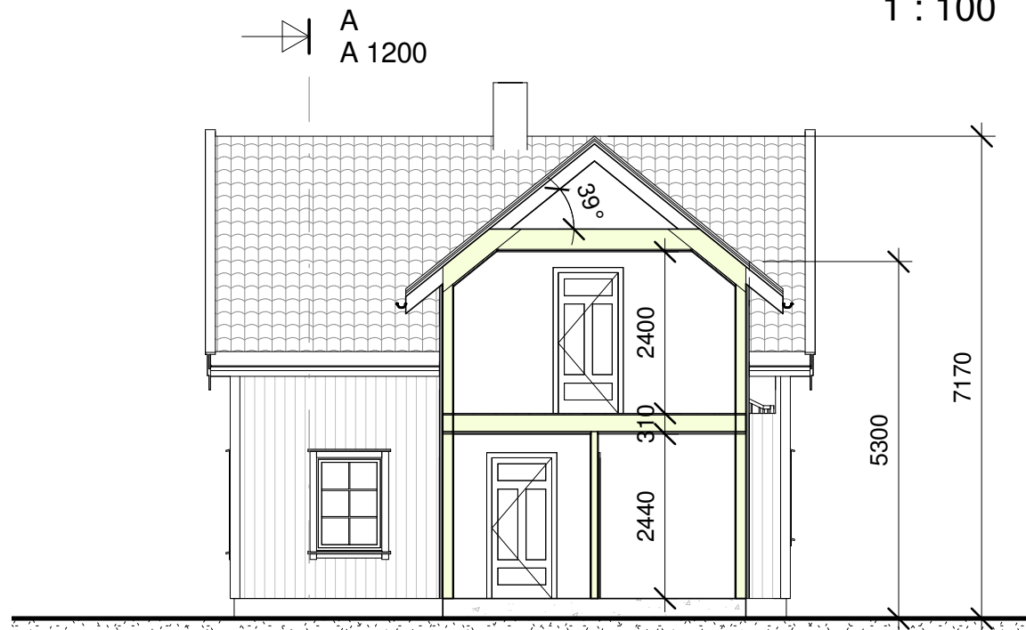
Snitt B-B 1 : 100
