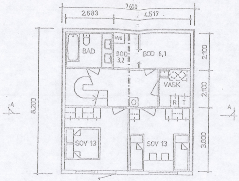
PLAN UNDERETASJE
