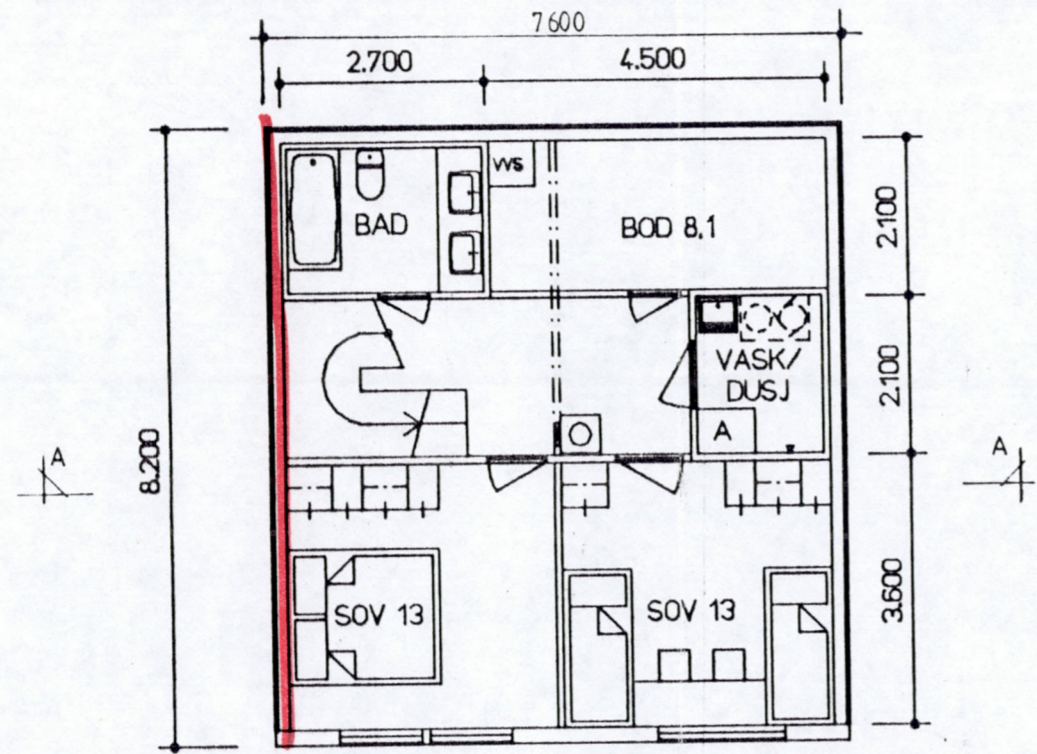
PLAN UNDERETASJE
