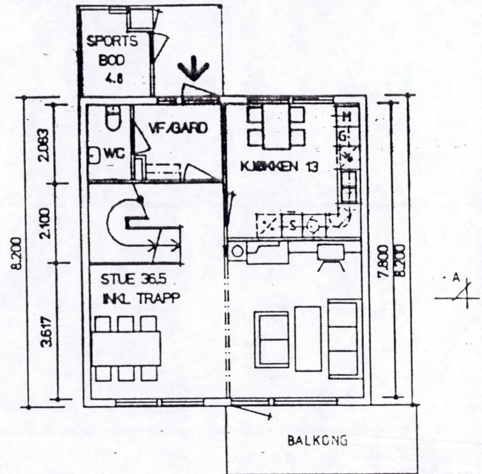
PLAN 1ETASJE
