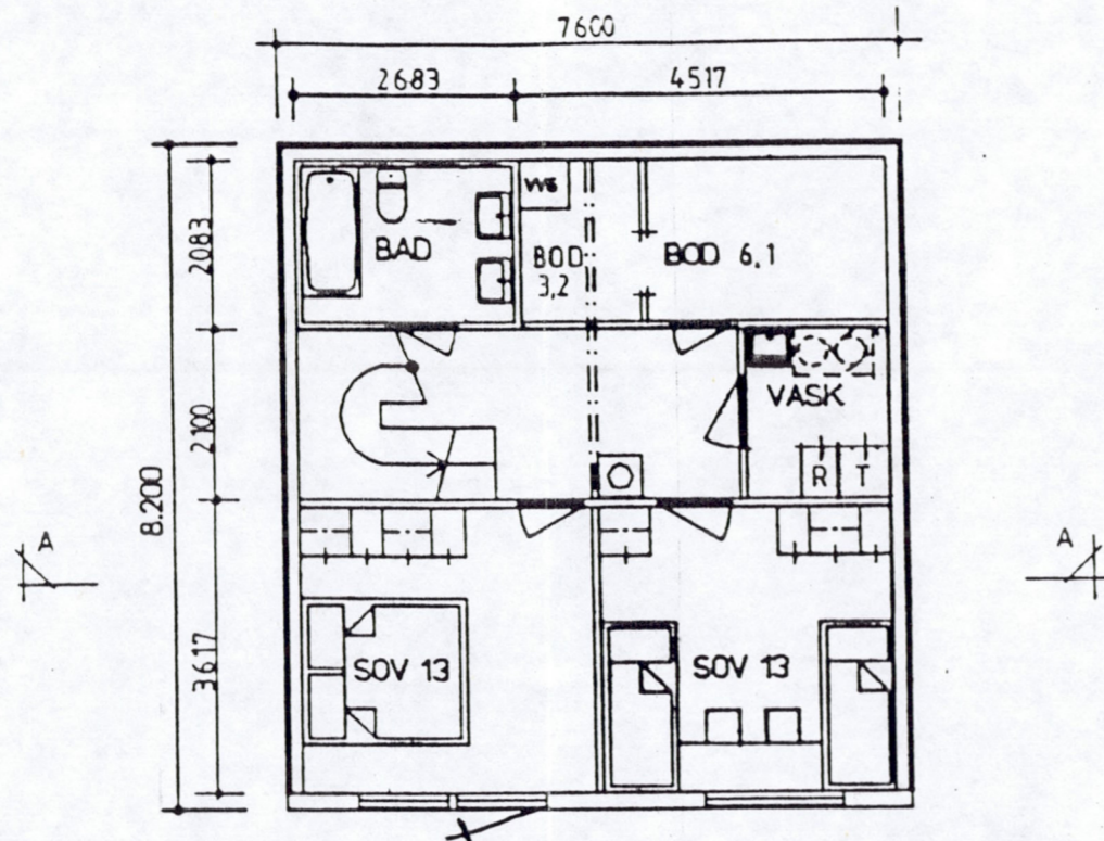
PLAN UNDERETASJE
