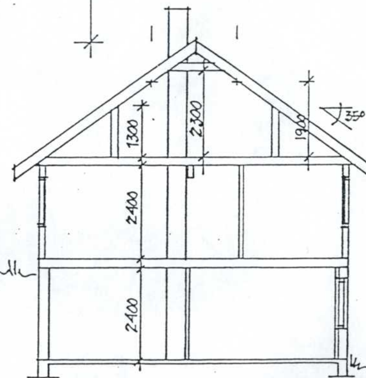
SNITT
