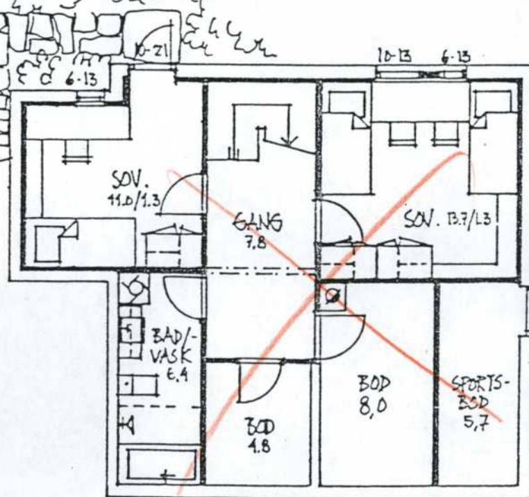
PLAN U. ET. TYPE A.1
