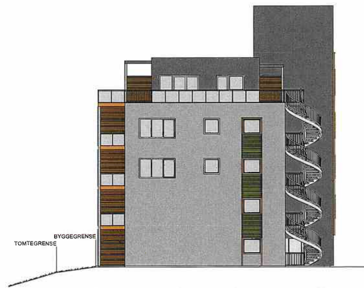
FASADE ØST, BYGG D
