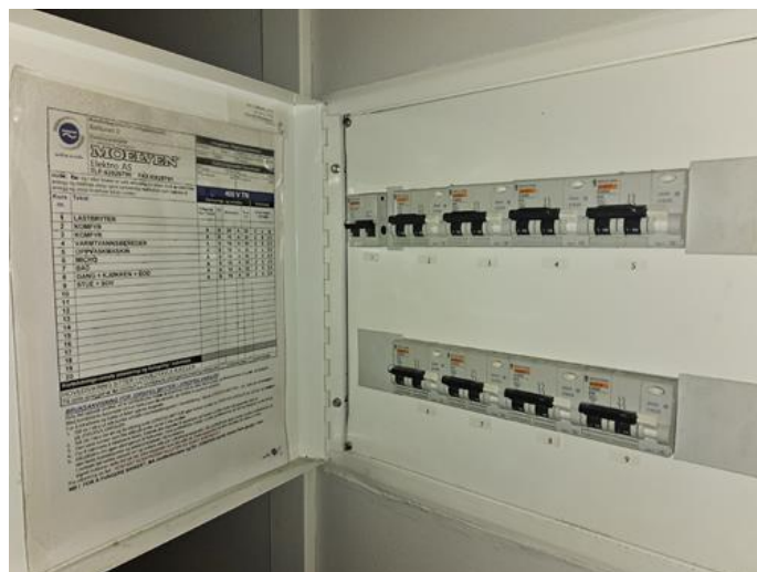
Elektrisk anlegg - [Sikringsskap og kursfortegnelse]
