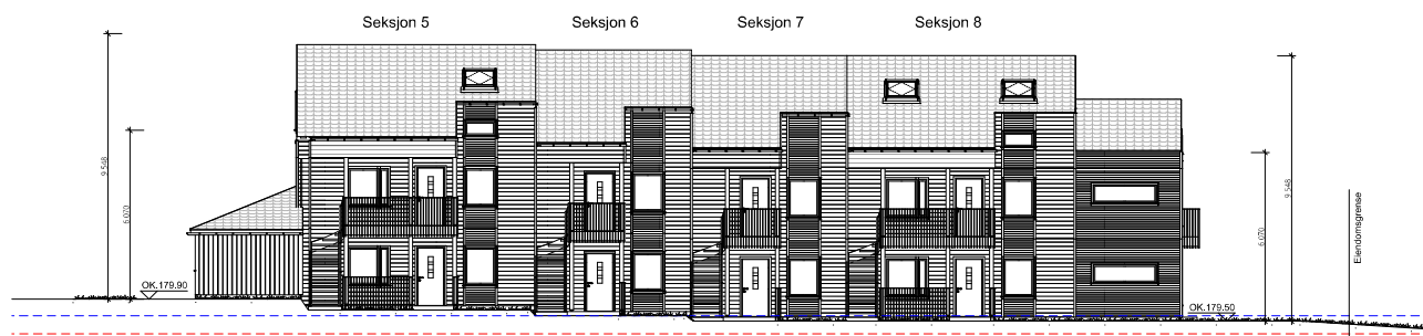
Fasade Øst
