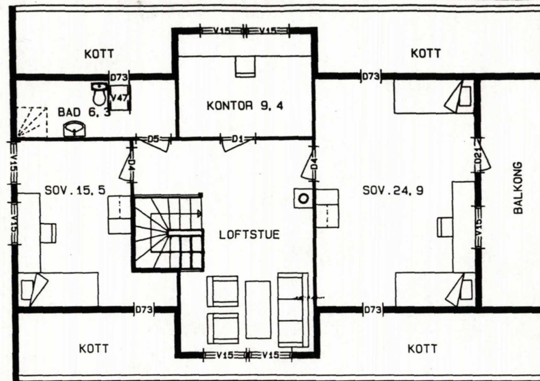
PLAN 2. ETASJE
