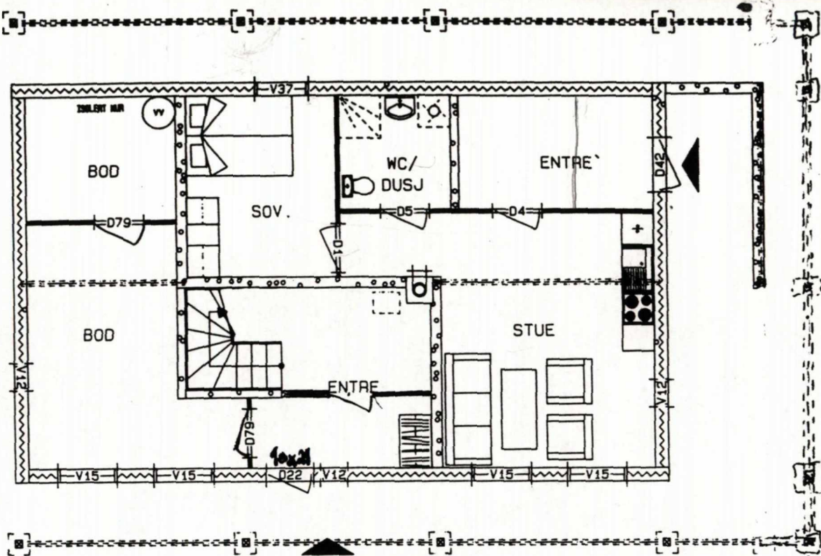
PLAN UNDERETASJE
