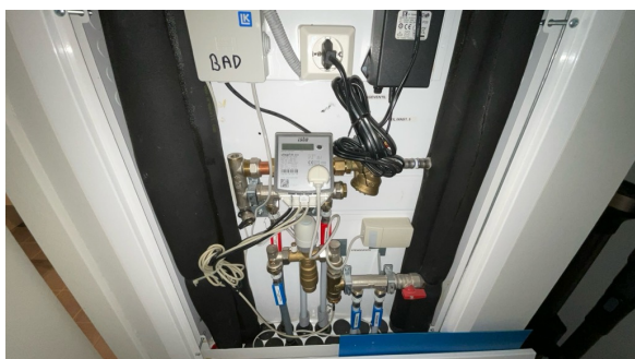
Fordelerskap for vannbåren radiatorvarme.
