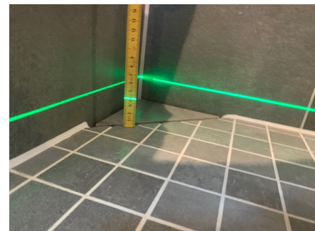
Avvik på fallforhold i et område i dusjsonen
