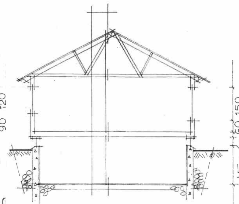
TVÆRSSNITT
