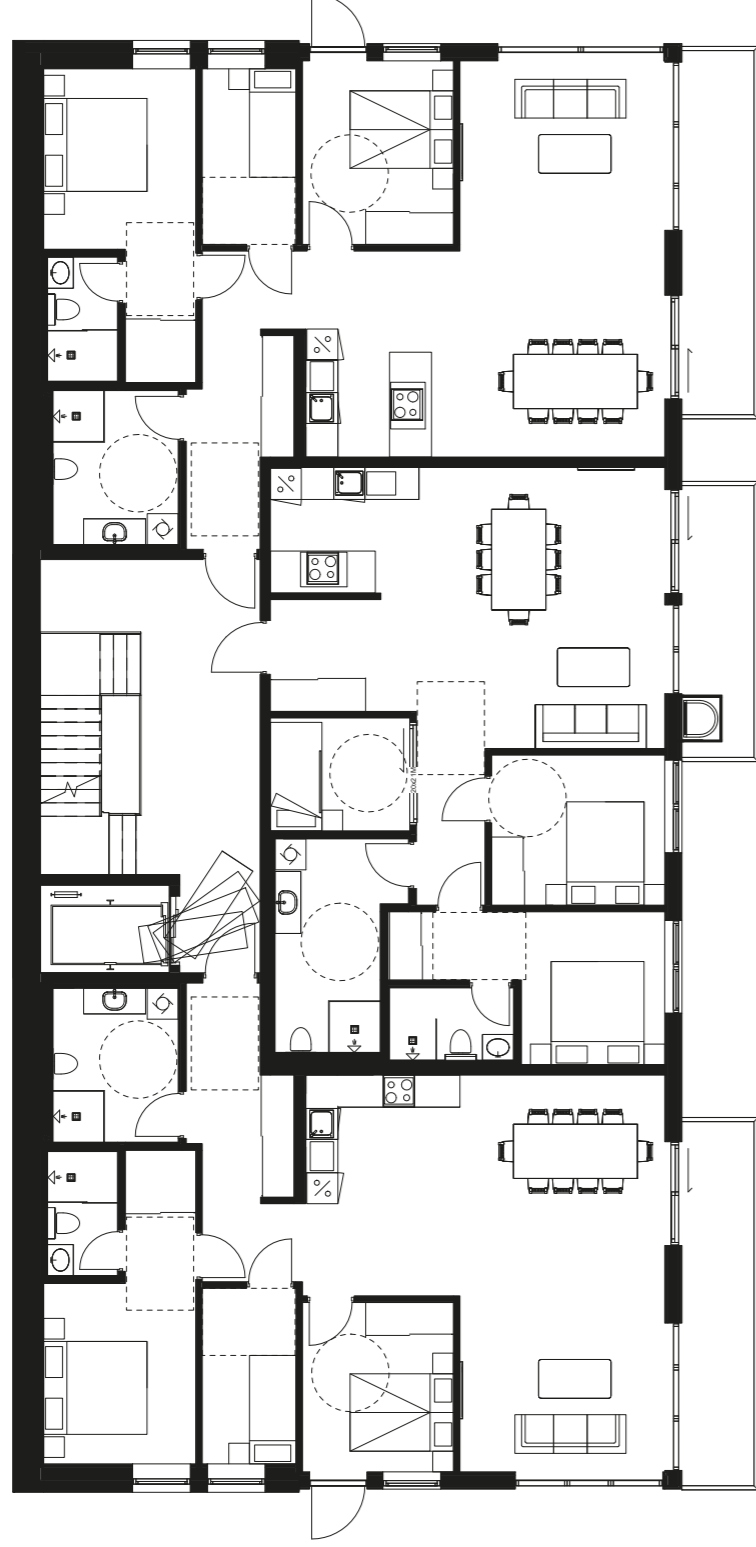
Plan 01 Salgstegning 1 : 100
