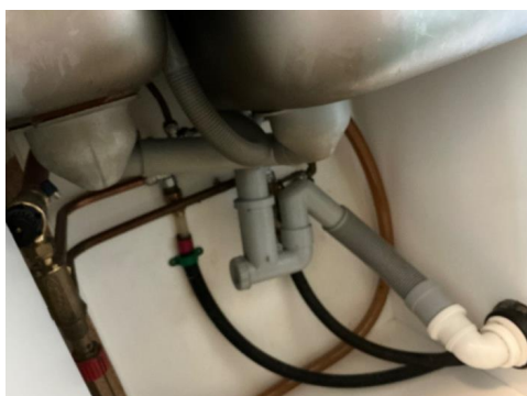
Avløp vask kjøkken
